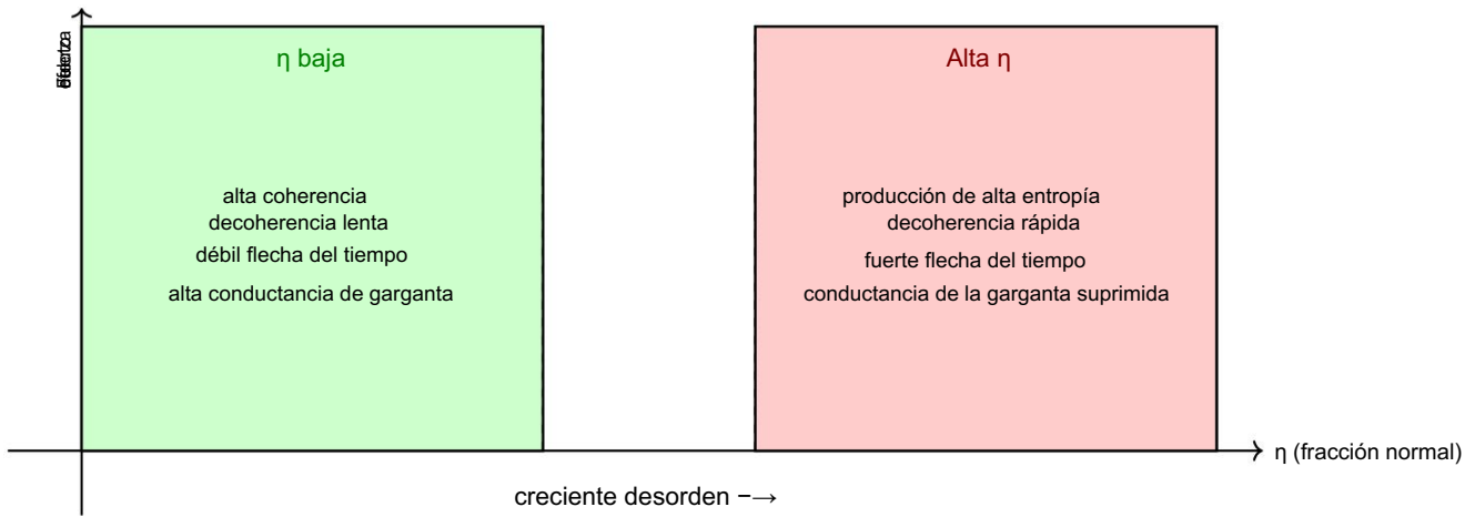
Figura 2: Consecuencias físicas de la fracción normal \eta . Las regiones de baja \eta son altamente coherentes y negentrópicas. Las regiones de alta \eta son entrópicas y temporalmente rígido. La dependencia exponencial de la conductancia de la garganta con respecto a \eta es una de las características dinámicas más importantes del modelo.
