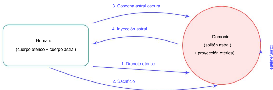
Figura 4: El ciclo parasitario de cuatro flujos. Los flujos 1 y 2 mantienen la presencia del demonio en el condensado hijo. Los flujos 3 y 4 sostienen su existencia natural en el condensado original. El sistema se autorrefuerza.
