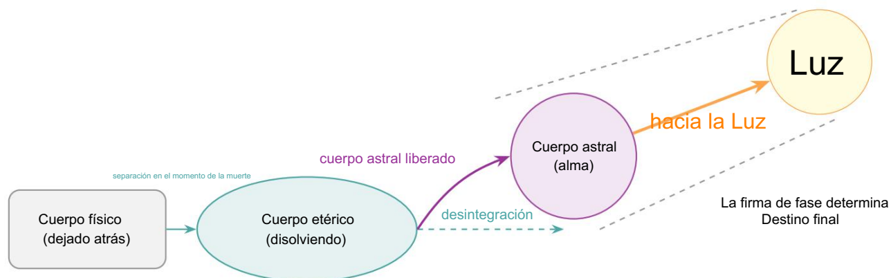
Figura 5: Dinámica post mortem en el modelo de condensado anidado. En la muerte biológica, el cuerpo físico permanece, el cuerpo etérico se disuelve gradualmente (liberando la energía almacenada) y el cuerpo astral se libera a través de la garganta personal ensanchada. Su fase acumulada La firma determina si se dirige hacia la "Luz" de baja \eta (regiones superiores) o hacia los dominios astrales inferiores de mayor \eta .
