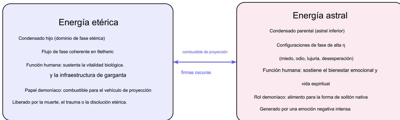
Figura 3: Las economías energéticas duales. La energía etérica (nivel hija) impulsa la proyección del demonio en nuestro espacio-tiempo, mientras que la energía astral (nivel padre) nutre su forma nativa de solitón de alta energía. Ambas están conectadas por flujos mutuos.
